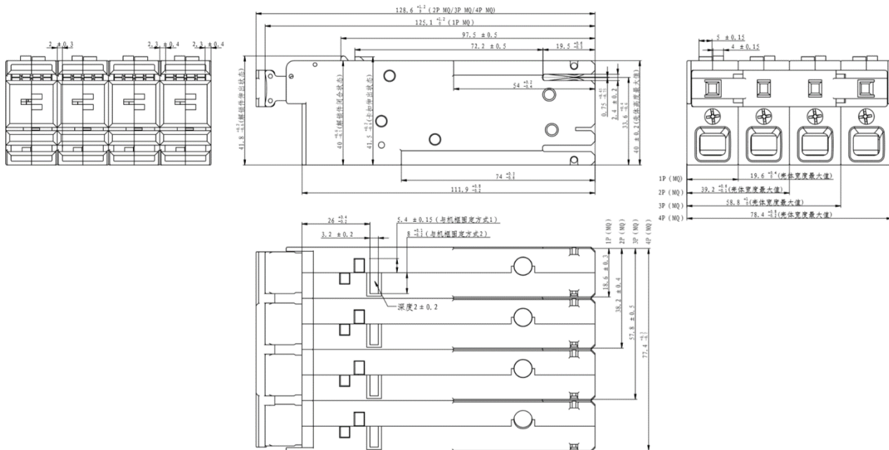
NDB6A-63H 1P (MQ) / 2P (MQ) / 3P (MQ) / 4P (MQ) 产品外形及安装尺寸
