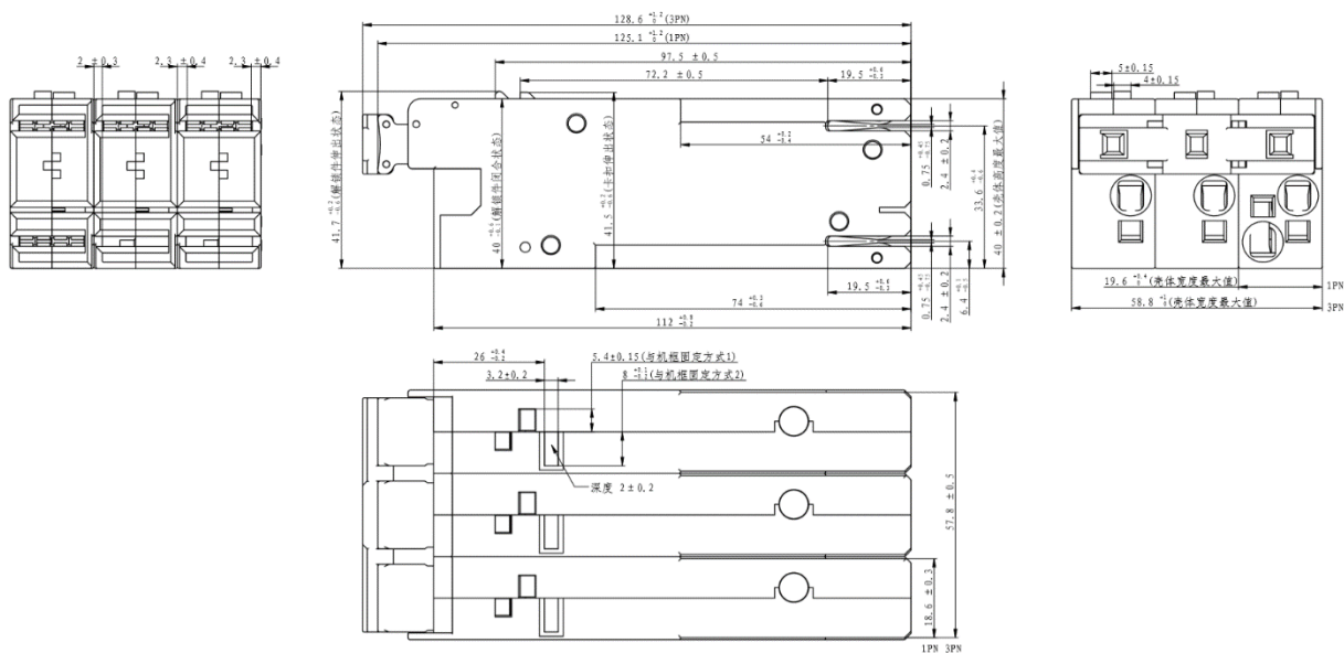
NDB6A-63H 1PN/3PN 产品外形及安装尺寸
