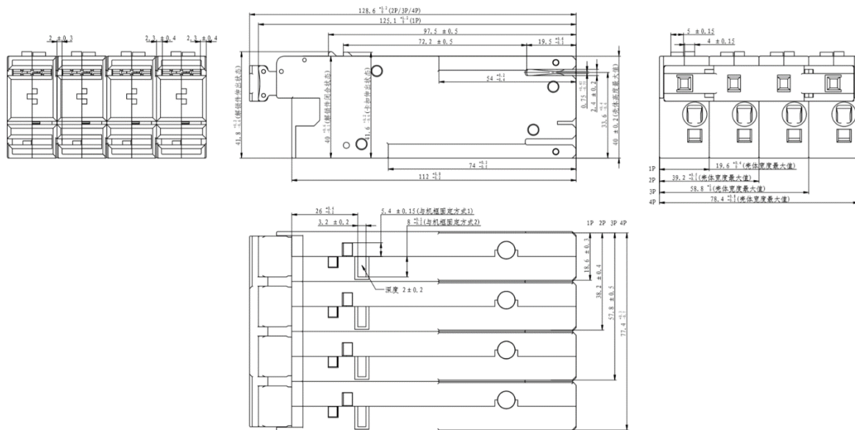
NDB6A-63H 1P/2P/3P/4P 产品外形及安装尺寸
